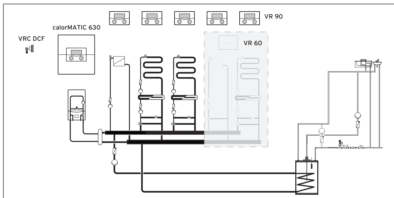
Рис. 3.1 Обзор системы
