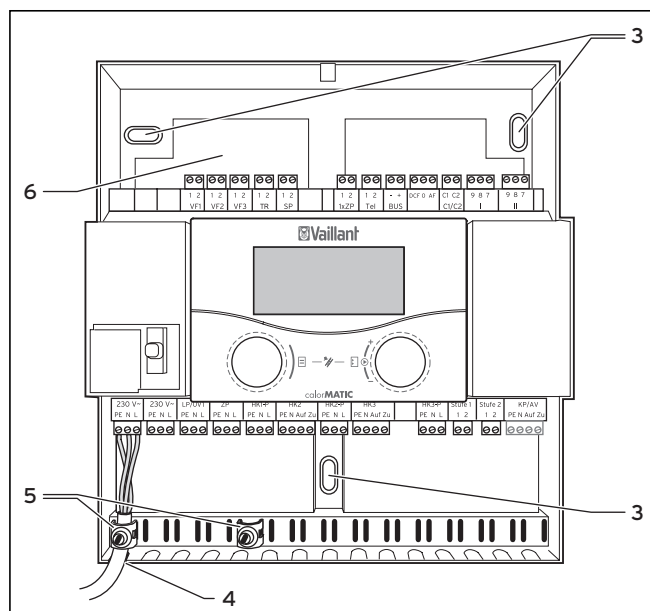
Рис. 4.3 Монтаж корпуса для настенного монтажа
