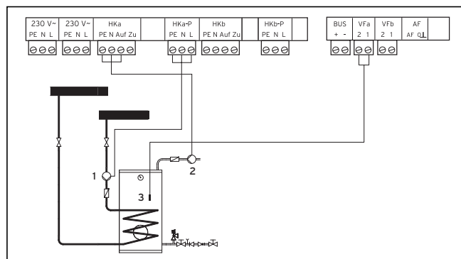
Рис. 5.3 Подключение смесительного контура в качестве контура нагрева накопителя
