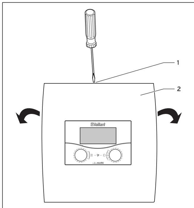
Рис. 4.2 Открытие корпуса для настенного монтажа
